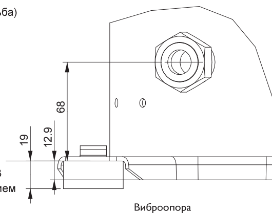
Виброопора
