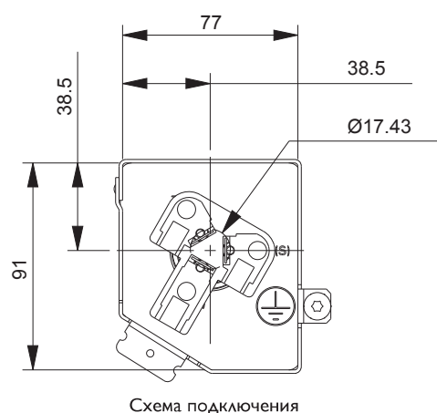
Схема подключения
